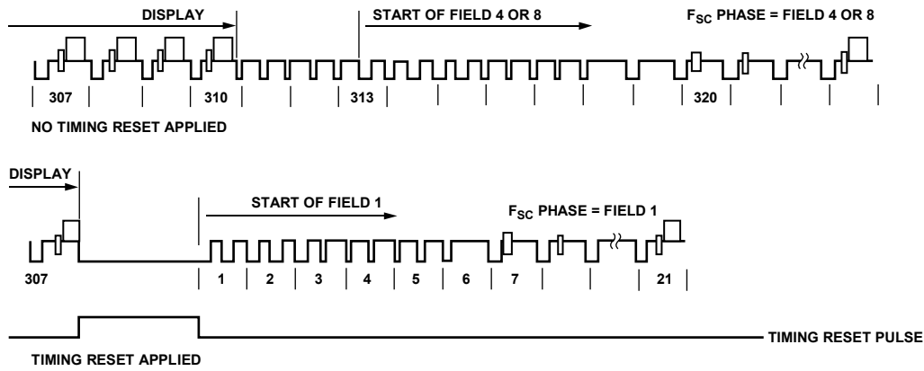
Figure 59. SD Timing Reset Timing Diagram (Subaddress 0x84, Bits[2:1] = 10)
